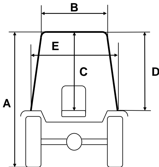
Cabina CLAAS NEXOS 230 LD Gommatura Post. Trattore 380/70 R.24
