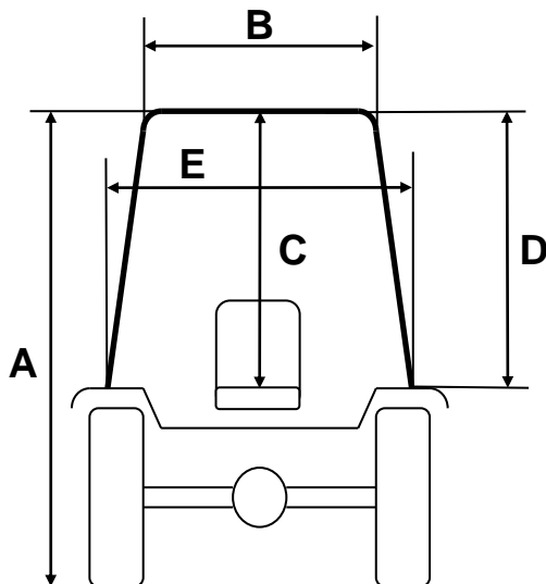
Cabina New Holland T4.80+BASSOTTO Stage V Gommatura Posteriore Trattore 360/70 R.20
