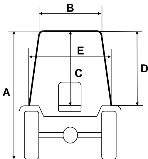
Cabina BCS VOLCAN SDT K105 RS Monodirezionale Gommatura Posteriore Trattore 360/70 R.20
