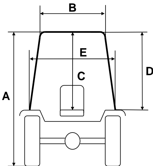
Cabina BCS VOLCAN SDT 850 RS Monodirezionale Gommatura Posteriore Trattore 320/70 R.24
