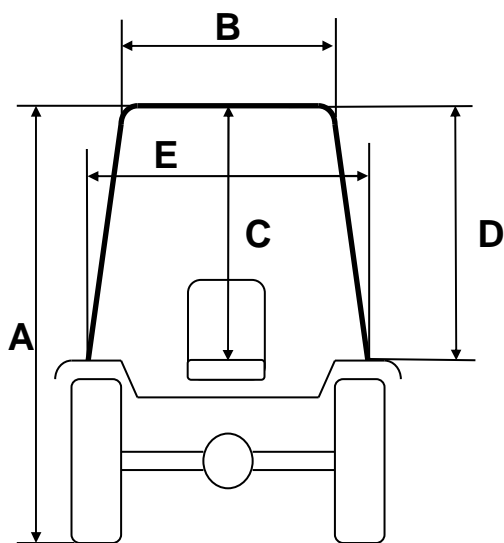
CABINA Carraro Antonio SN 6500 V Gommatura Trattore 280/70 R.18
